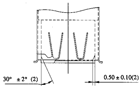
图3 连接插座（USB A系列）的结构及尺寸一
