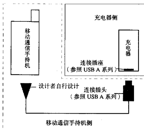
图2 连接结构示意图二
