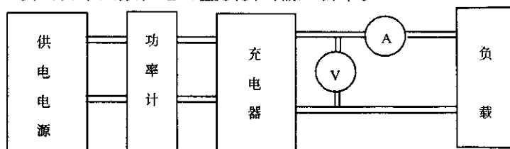
图9 充电器平均效率测试连接图
