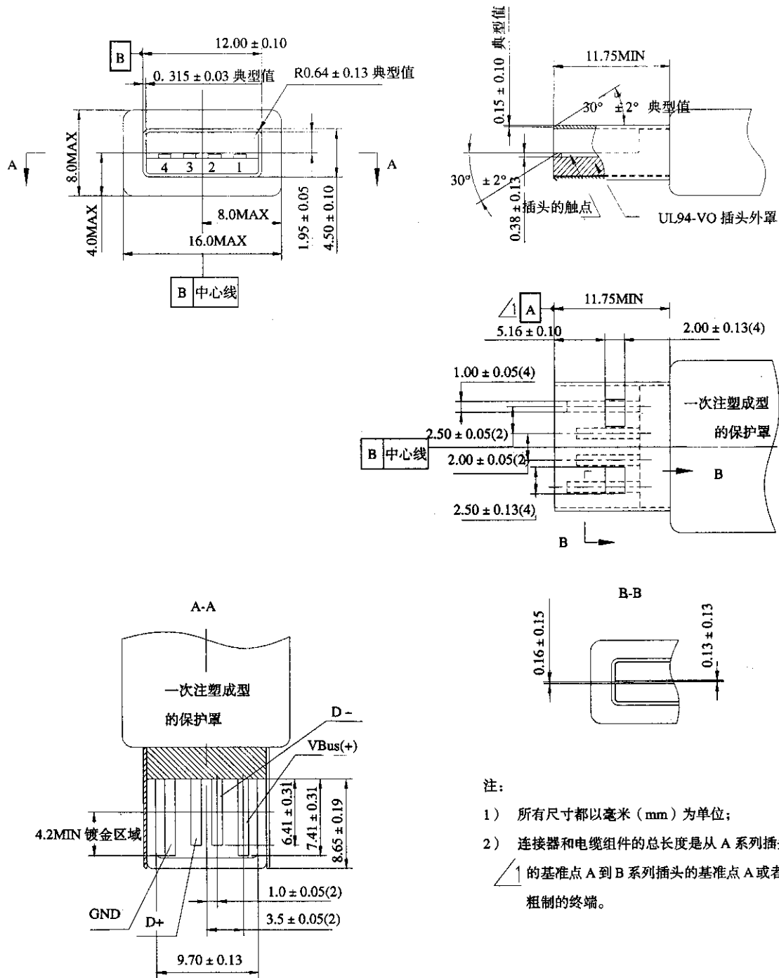
图4 连接插头 (参照 USB A 系列) 的结构和尺寸二
