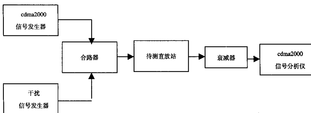
图 12 阻塞的测试配置
