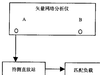
图5 输入/输出电压驻波比测试配置
