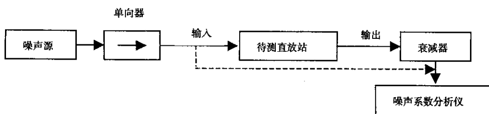
图6 噪声系数测试配置
