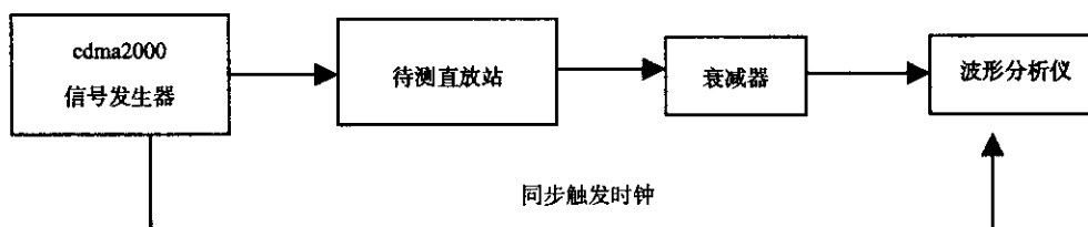
图9 波形质量因数测量配置
