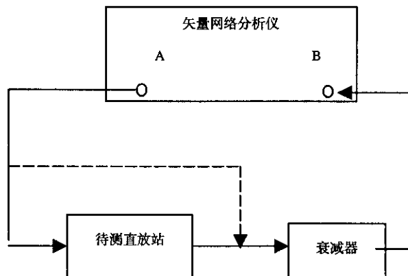
图4 传输时延测试配置
