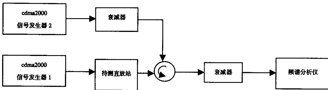
图11 输出互调的测试配置
